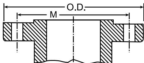
Flange
